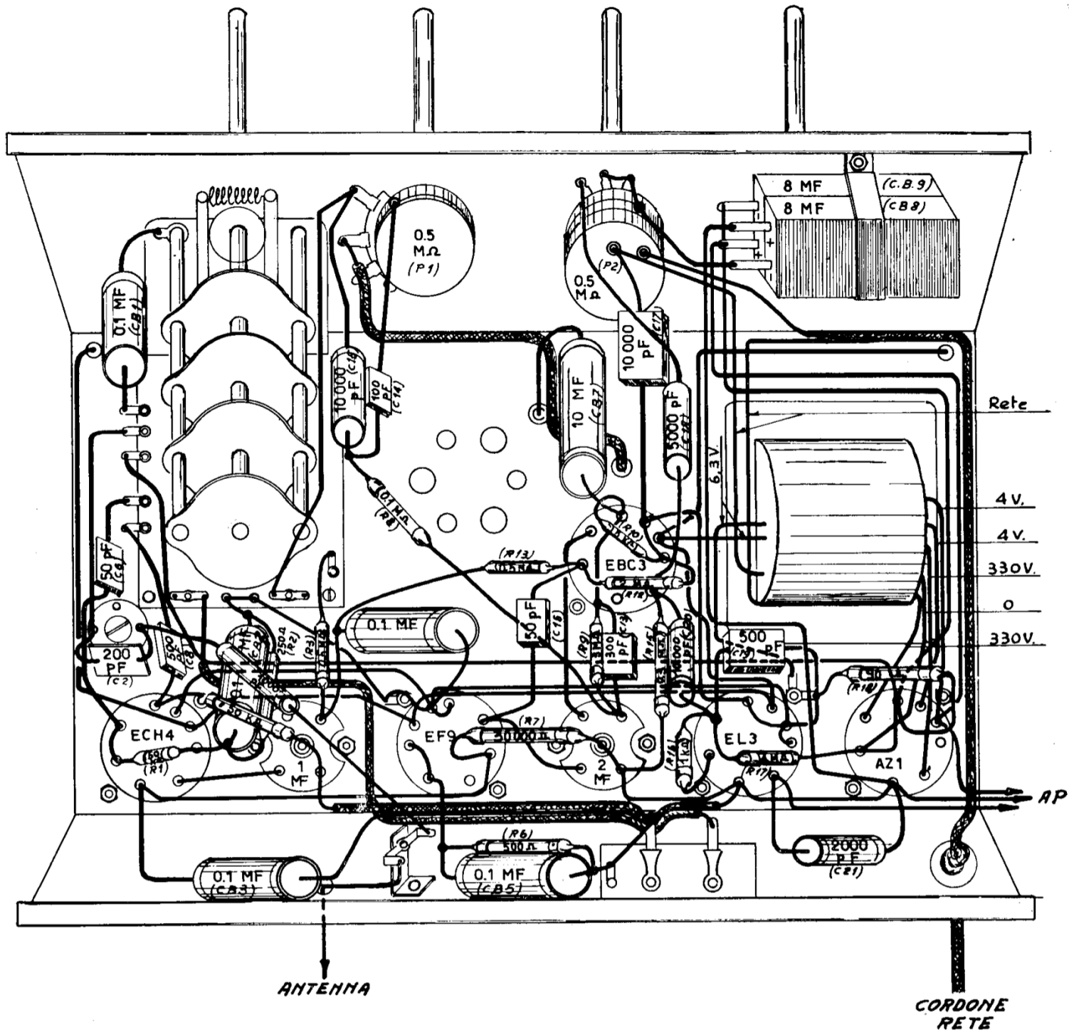
RICEVITORE ULTRA S 53 - Vista inferiore
